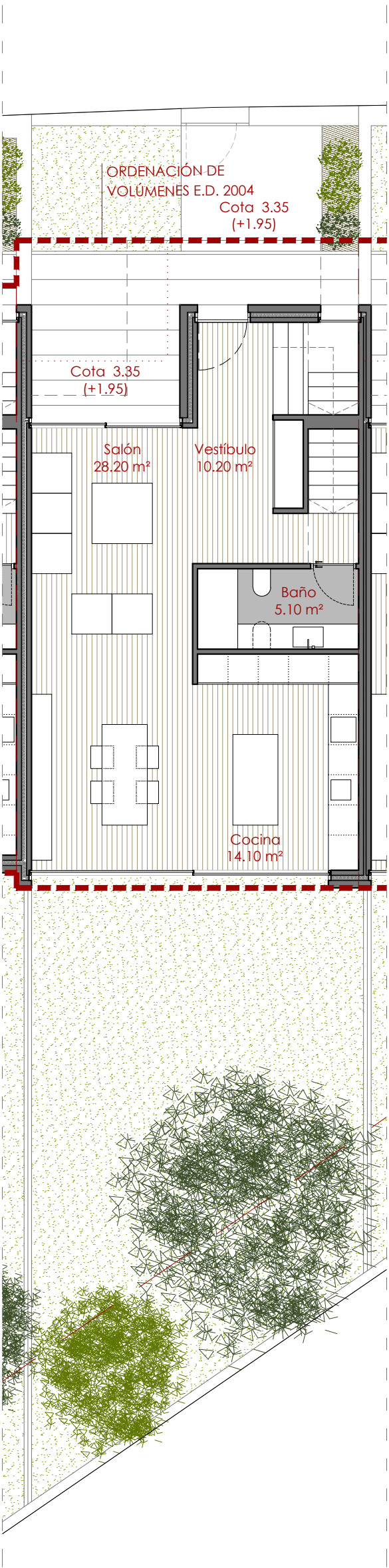
Planta baja
